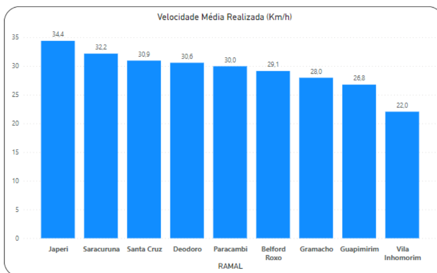
Gráfico 3.69 SuperVia – Velocidade Média Realizada
